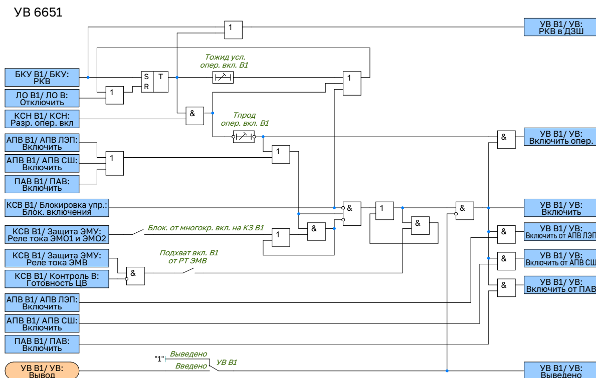
Рисунок 2.81 – Функциональная схема управления выключателем В1
