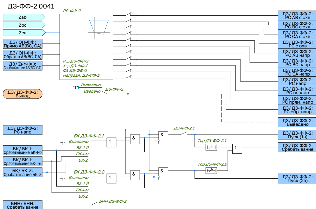
Рисунок 2.33 – Функциональная схема логики ДЗ-ΦΦ-2
