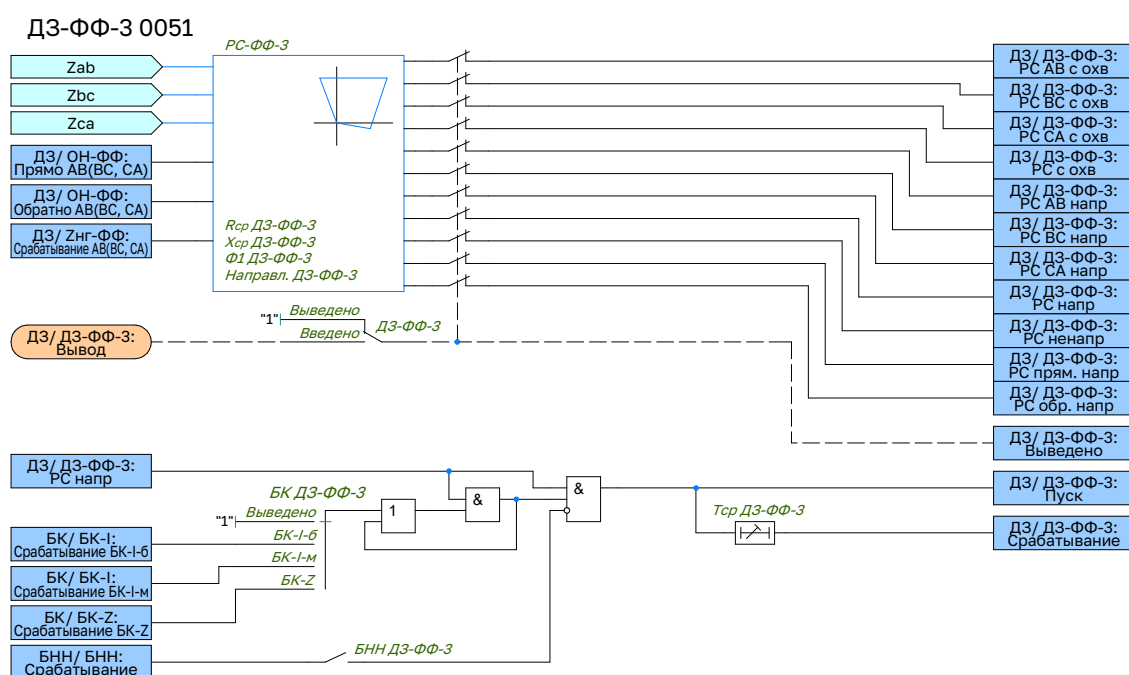
Рисунок 2.34 – Функциональная схема логики ДЗ-ΦΦ-3
