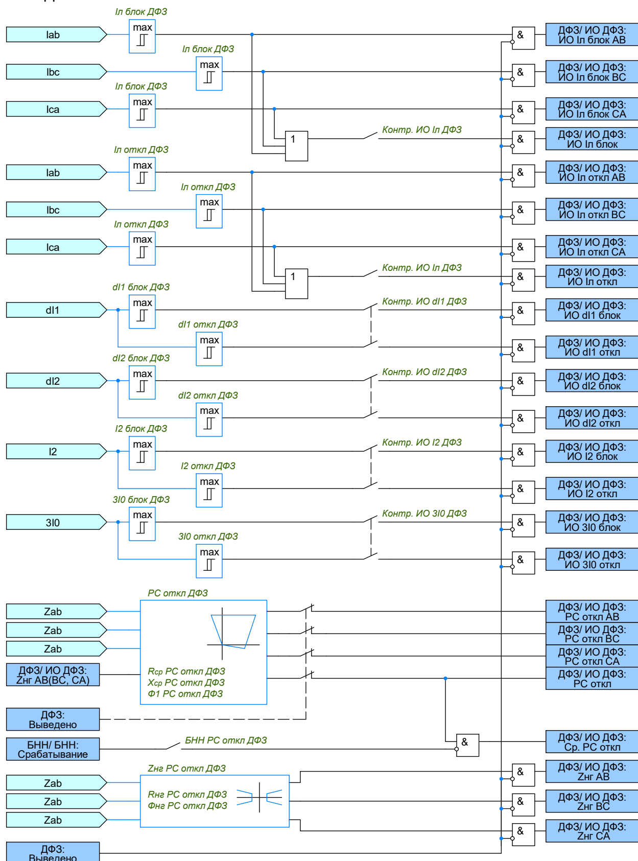
Рисунок 2.2 – Измерительные органы ДФЗ
