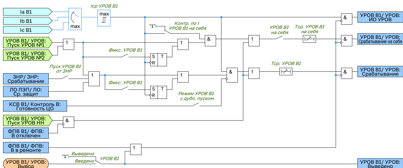
Рисунок 2.66 – Функциональная схема логики УРОВ В1
